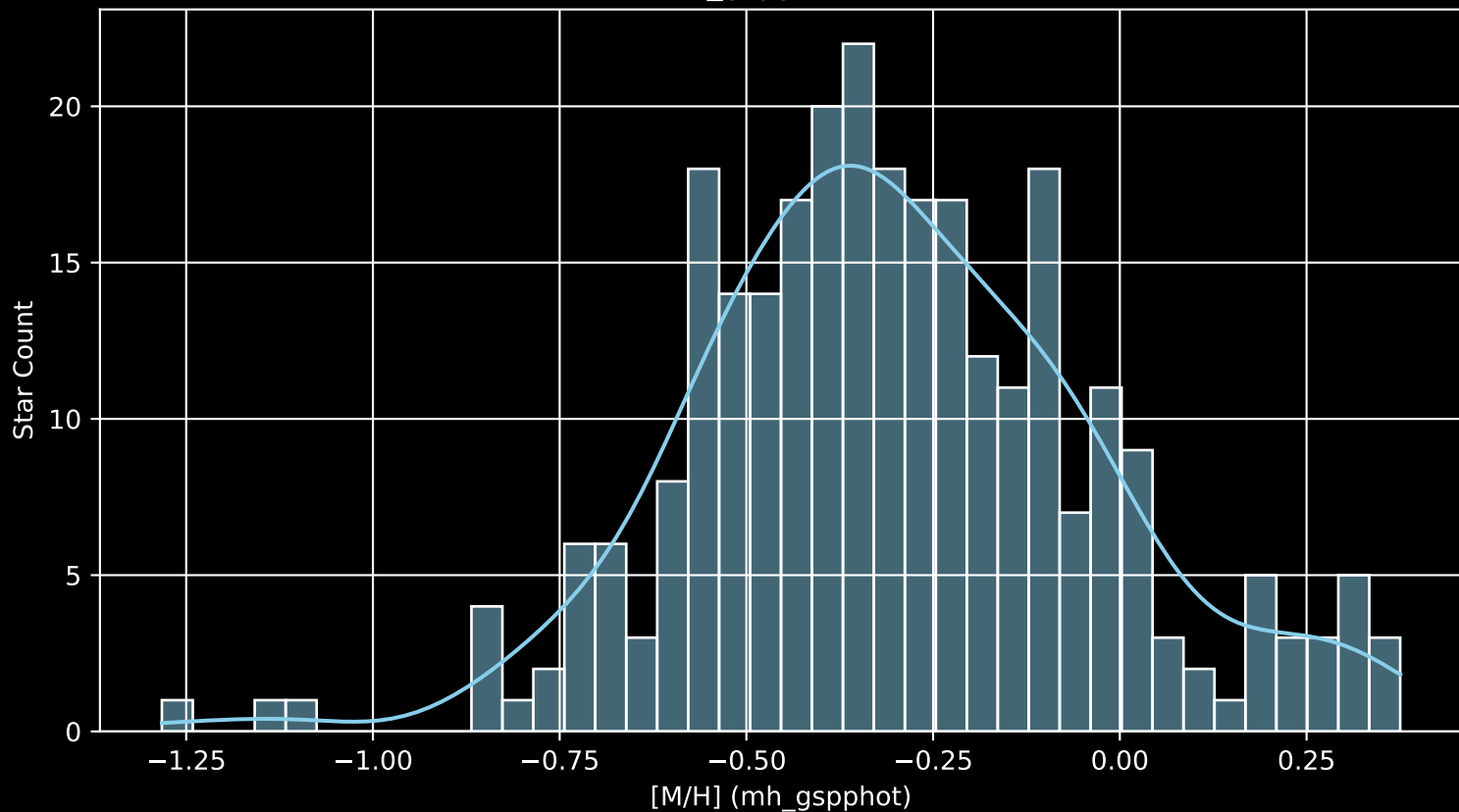
GALAH DR4 Field: [1832] [M/H] (mh_gspphot) (n= 283)
