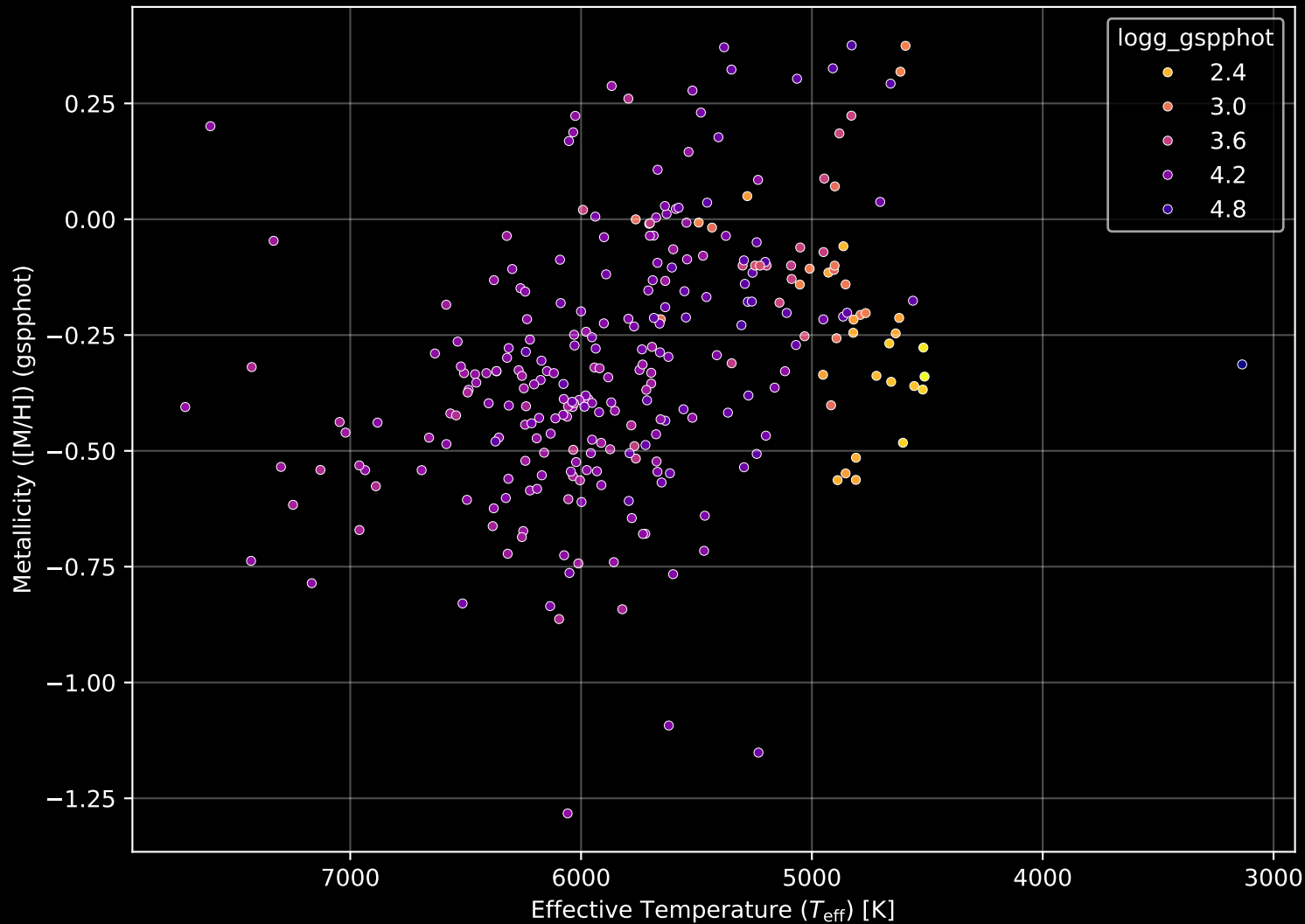
GALAH DR4 Field: [1832] Stellar Population Parameters (n= 283)
