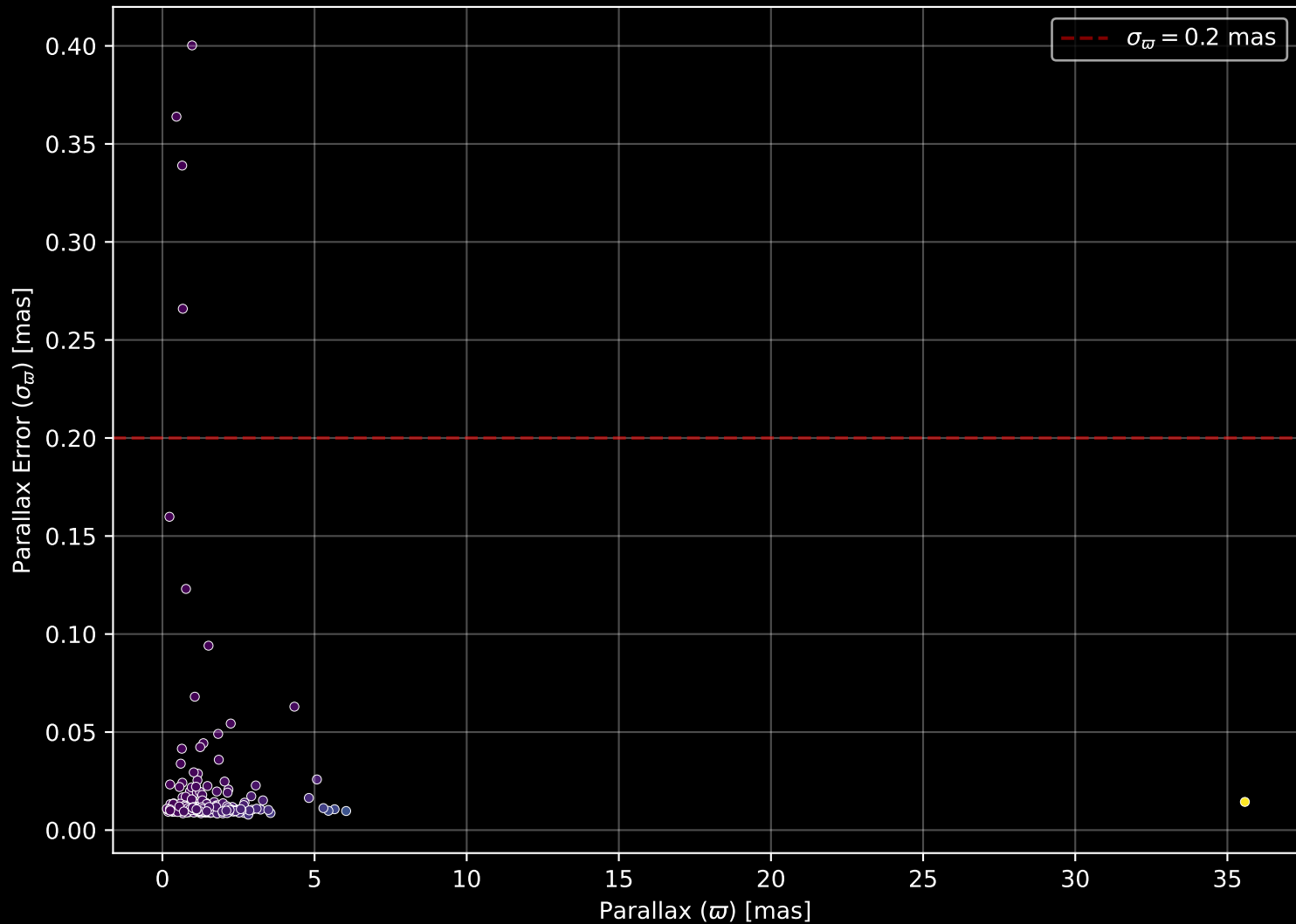
GALAH DR4 Field: [1832] Parallax Quality (n= 283)
