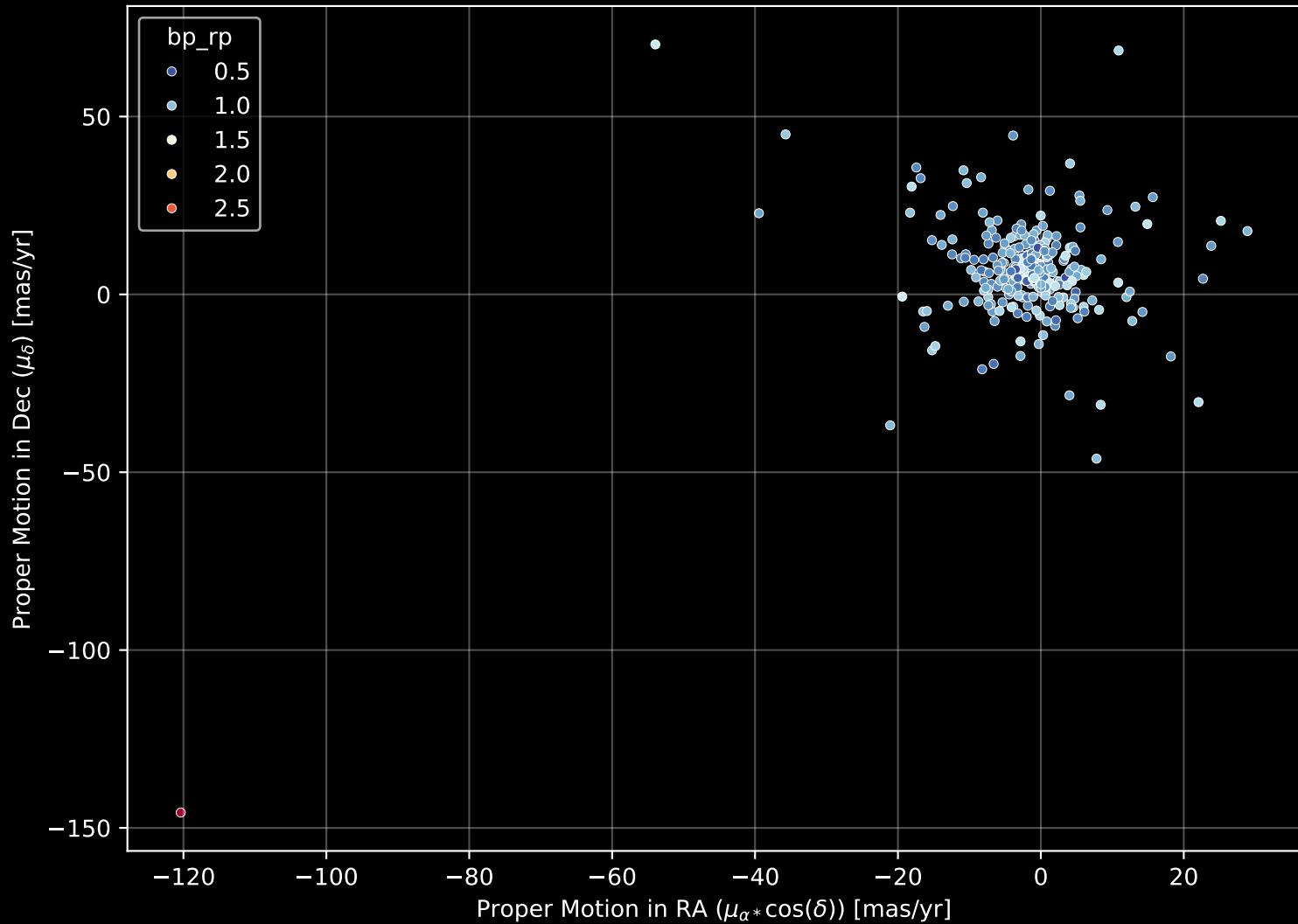
GALAH DR4 Field: [1832] Proper Motion Diagram (n= 283)
